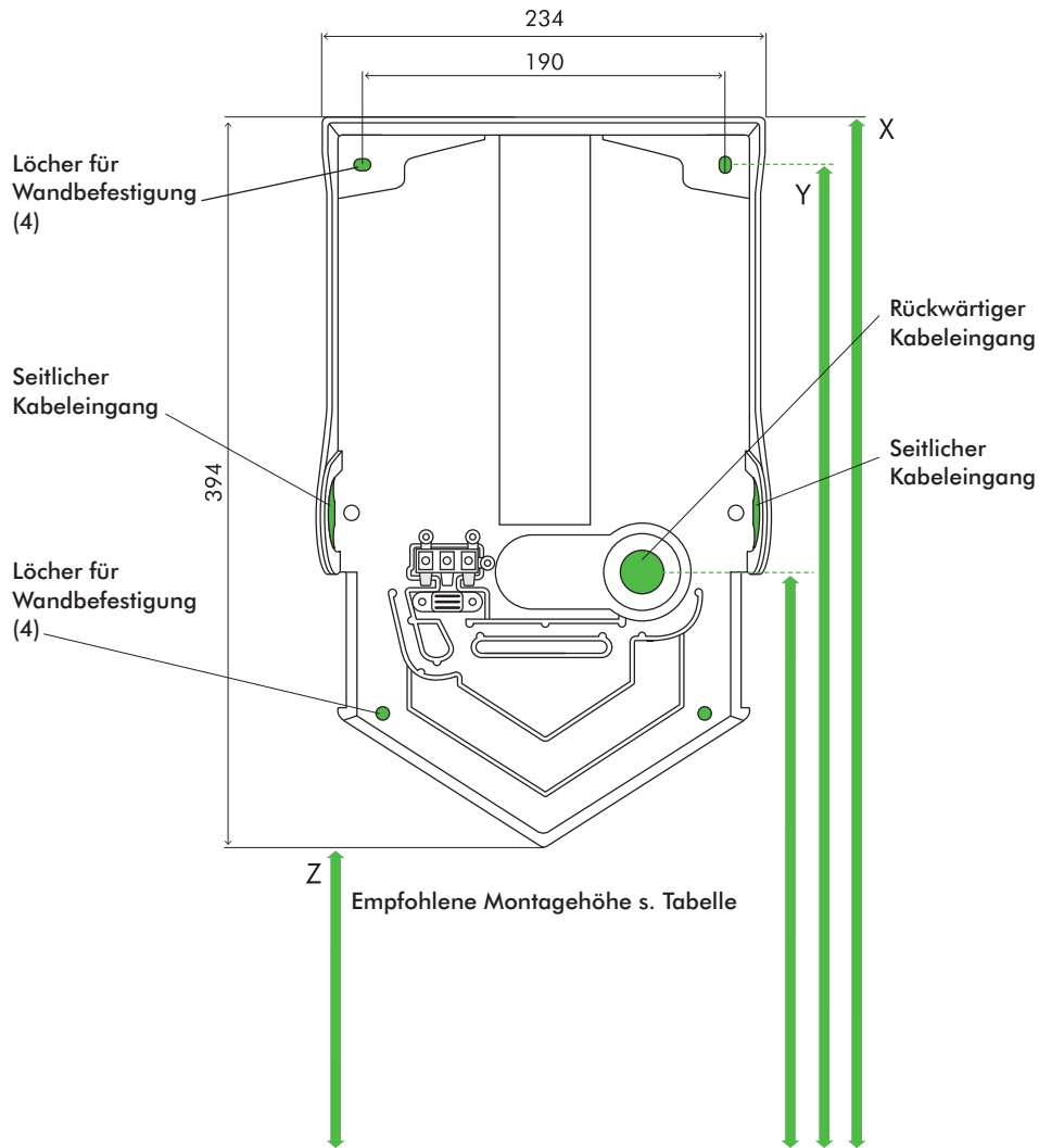
RÜCKANSICHT
