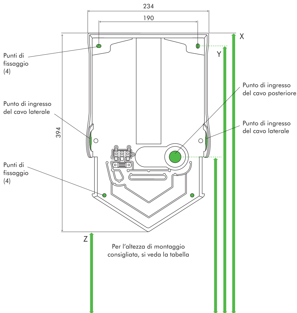
VISTA POSTERIORE
